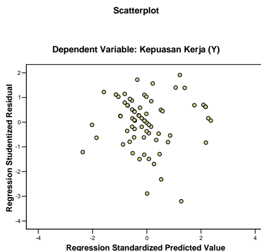
Gambar 3. Grafik Scatterplot
