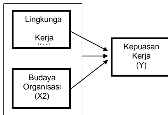
Gambar 1. Kerangka berfikir
