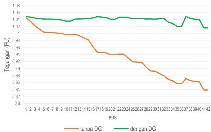
Gambar 6. Profil tegangan tanpa dan dengan dua DG
