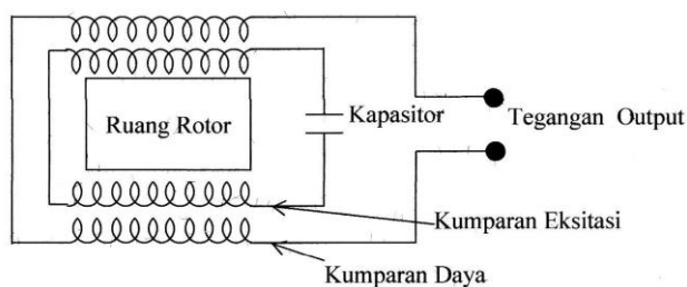
Gambar 2. Konstruksi Kumparan Stator
