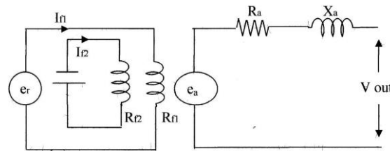
Gambar 5. Rangkaian ekivalen Generator Induksi.
