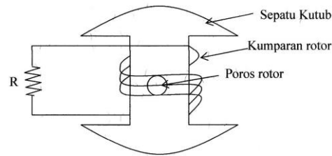
Gambar 3. Bentuk Rotor
