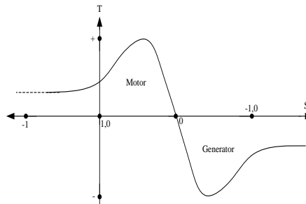
Gambar 1. Daerah kerja mesin induksi.
