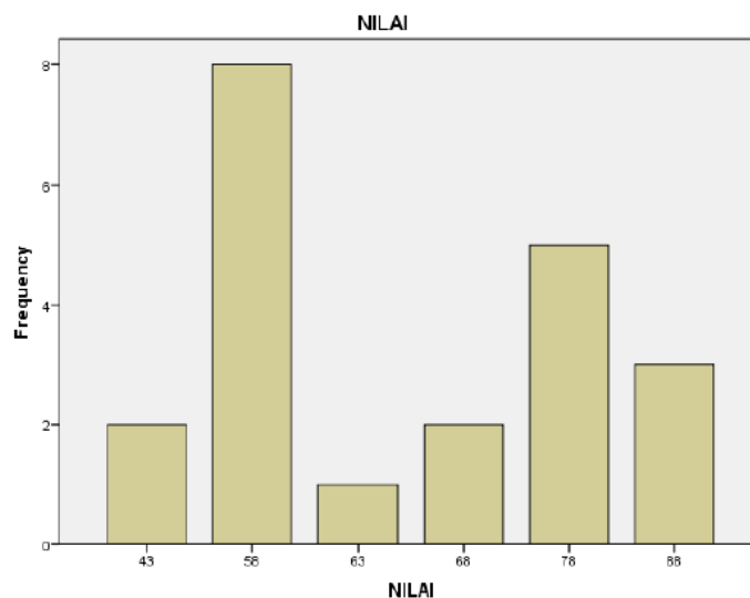
Gambar 2. Diagram Batang Data Nilai Siswa Kelas Kontrol
