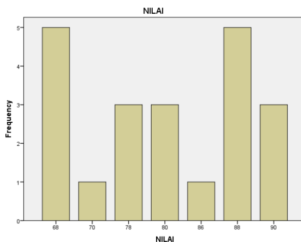
Gambar 1. Diagram Batang Data Nilai Siswa Kelas Eksperimen
