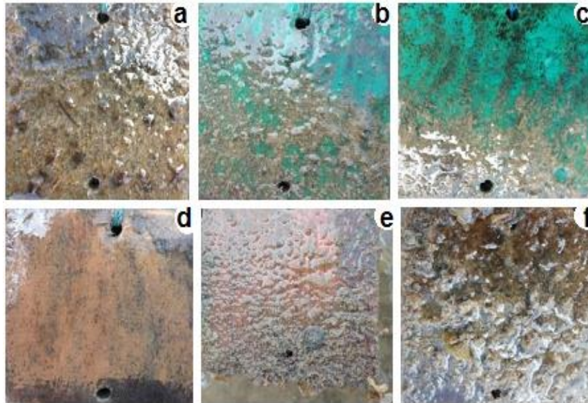
Gambar 1. Plat kayu yang direndam dalam laut selama 8 minggu. a) EDRA; b) cat kayu; c) EDRA+cat kayu; d) EDRA+Vernis; e) Vernis; f) tanpa pengecatan.
