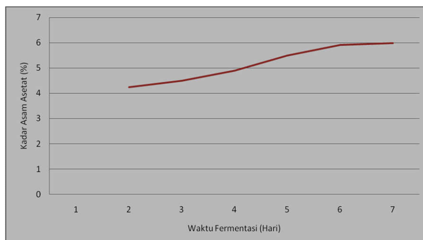
Gambar 1. Hubungan antara kadar asam asetat dengan waktu fermentasi pada penambahan induk cuka sebanyak 15%
