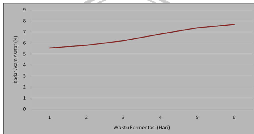
Gambar 3. Hubungan antara kadar asam asetat dengan waktu fermentasi pada penambahan induk cuka sebanyak 23%
