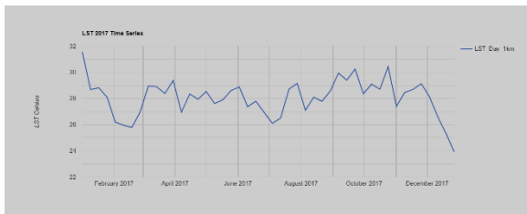
Gambar 13. Grafik Suhu Permukaan Tanah Tahun 2017
