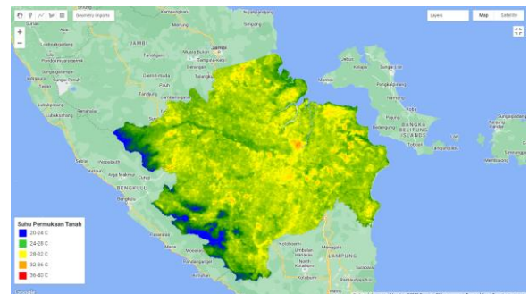
Gambar 8. Suhu Permukaan Tanah Tahun 2020
