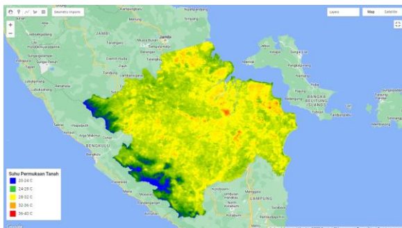
Gambar 4. Suhu Permukaan Tanah Tahun 2016
