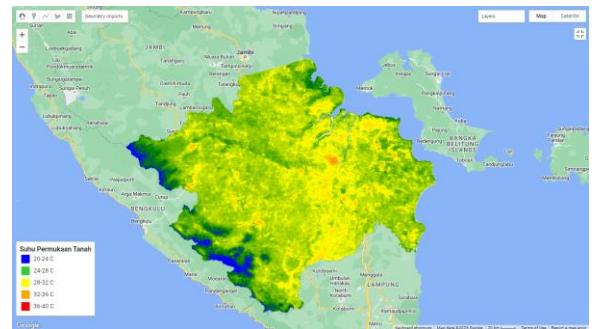
Gambar 9. Suhu Permukaan Tanah Tahun 2021
