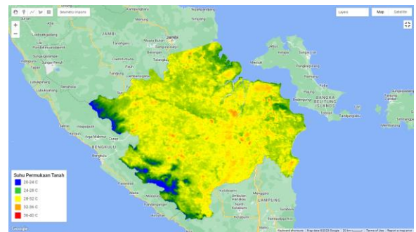
Gambar 7. Suhu Permukaan Tanah Tahun 2019
