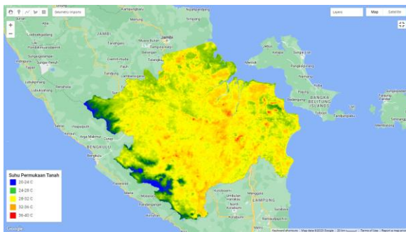
Gambar 3. Suhu Permukaan Tanah Tahun 2015
