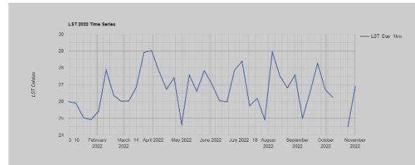
Gambar 18. Grafik Suhu Permukaan Tanah Tahun 2022
