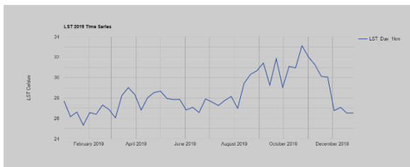
Gambar 15. Grafik Suhu Permukaan Tanah Tahun 2019
