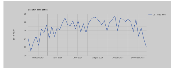
Gambar 17. Grafik Suhu Permukaan Tanah Tahun 2021
