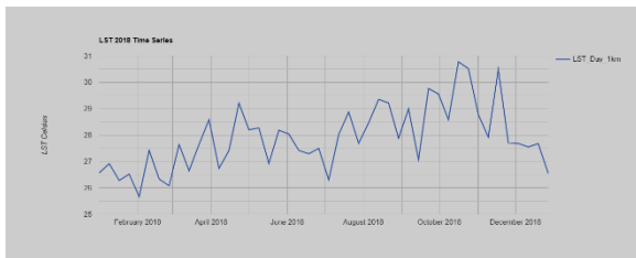
Gambar 14. Grafik Suhu Permukaan Tanah Tahun 2018
