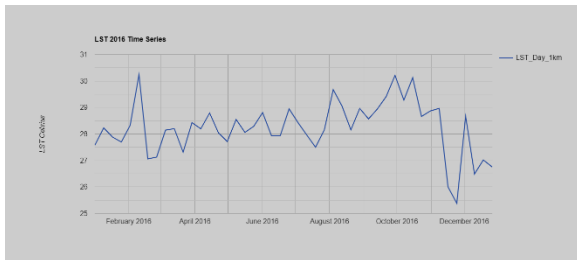
Gambar 12. Grafik Suhu Permukaan Tanah Tahun 2016
