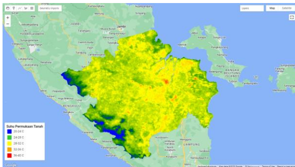
Gambar 5. Suhu Permukaan Tanah Tahun 2017
