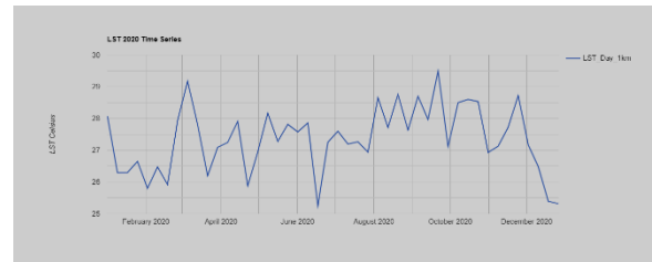
Gambar 16. Grafik Suhu Permukaan Tanah Tahun 2020
