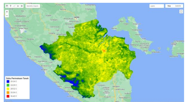
Gambar 10. Suhu Permukaan Tanah Tahun 2022
