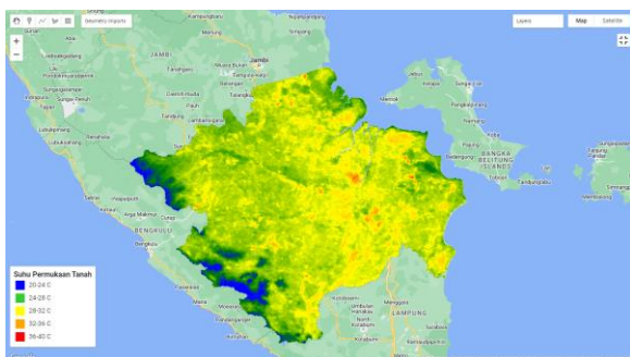
Gambar 6. Suhu Permukaan Tanah Tahun 2018
